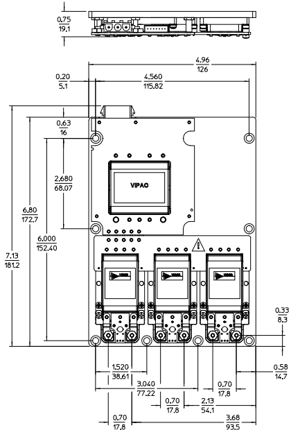
Configuration MVC-E / MVX-E
